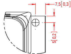
DETALHE A ESCALA 1 : 1
